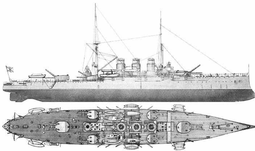
Броненосный крейсер I-го ранга "Рюрик", Российского Императорского Флота
